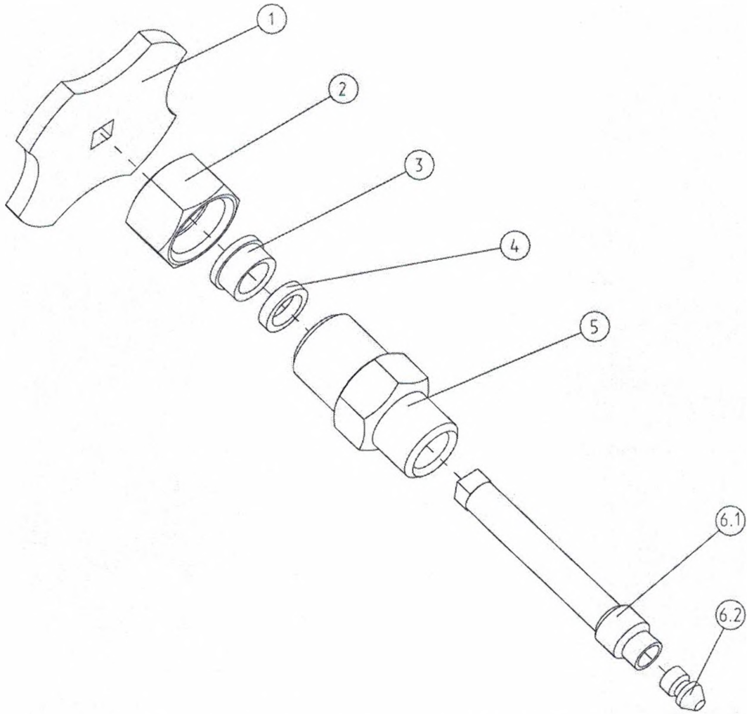
Рисунок 9 - Вентиль игольчатый КС-10.02.00.000А
