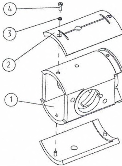
Рисунок 15 - Крейцкопф АФНИ.304516.001
