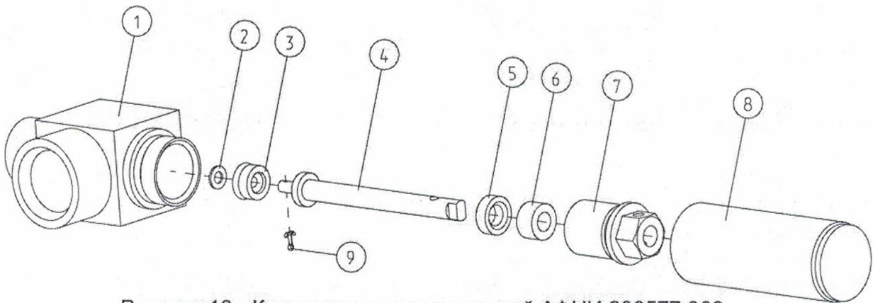
Рисунок 16 - Клапан предохранительный АФНИ.306577.002
