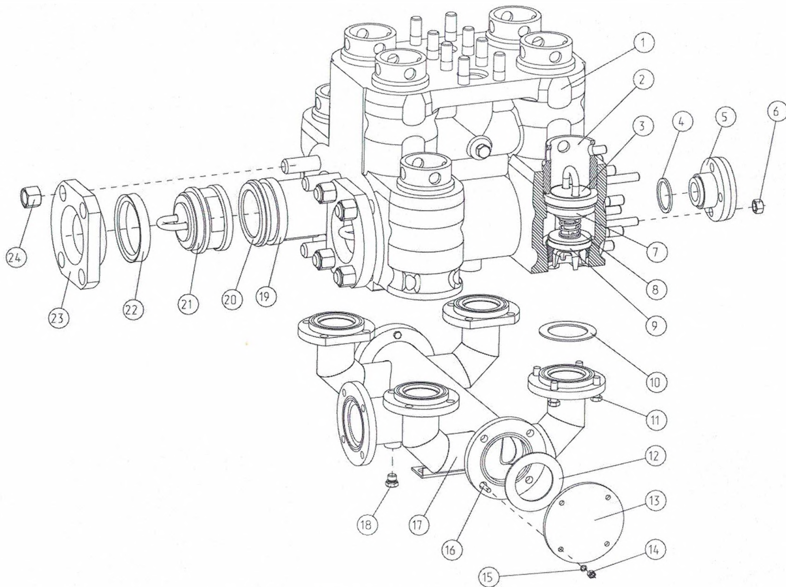
Рисунок 10 - Гидравлическая часть АФНИ.306555.001-02
