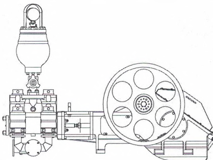
Рисунок 2 - Насос НБ-125ИЖ. Исполнение АФНИ.063168.004-28
