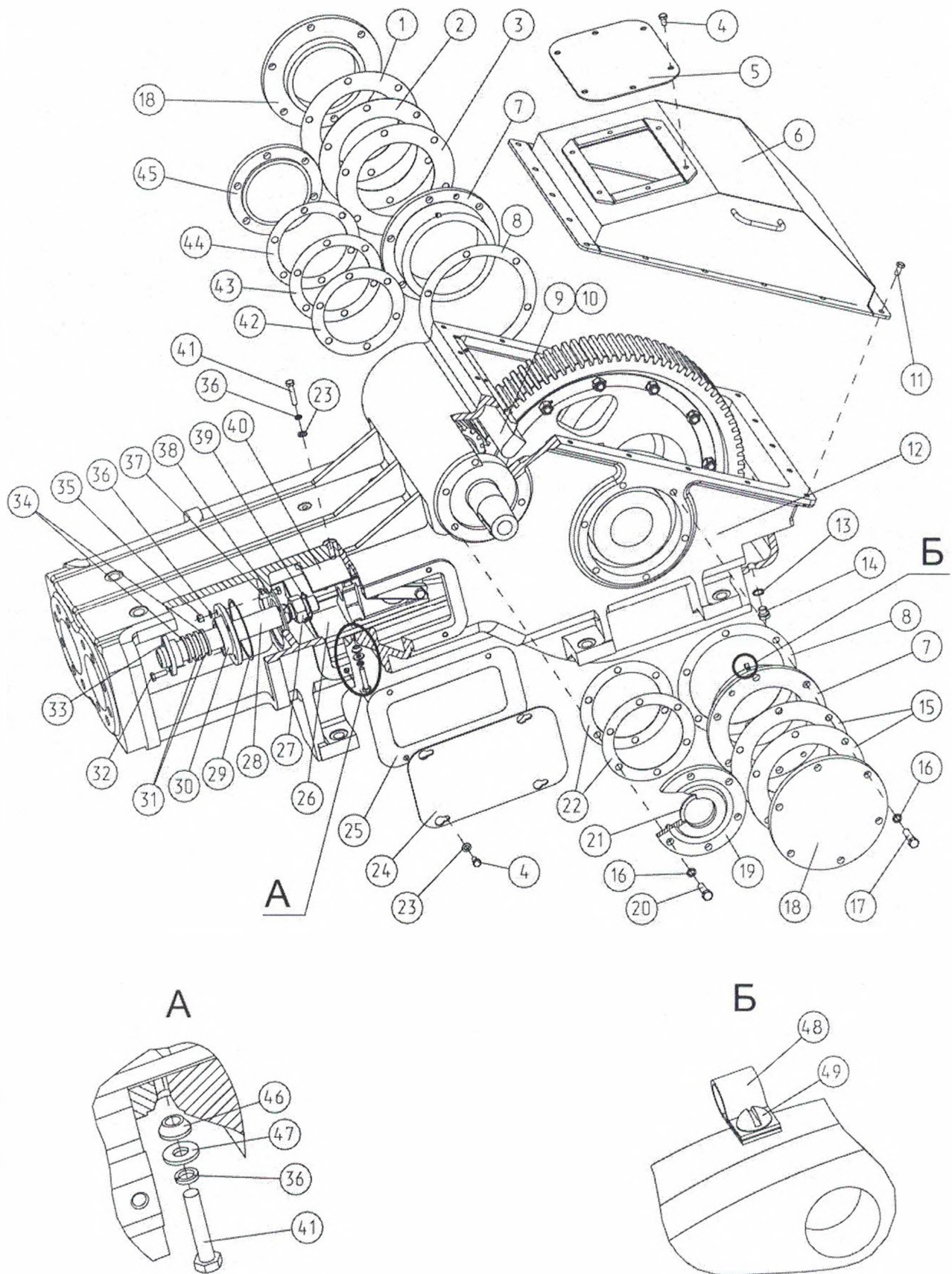
Рисунок 13а - Часть приводная НБ125.01.000
