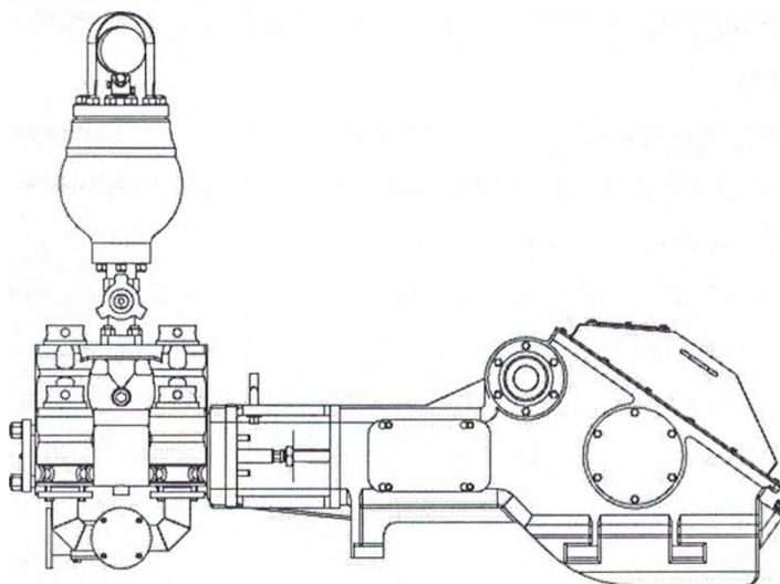
Рисунок 1 - Насос НБ-125ИЖ. Исполнение АФНИ.063168.004-27
