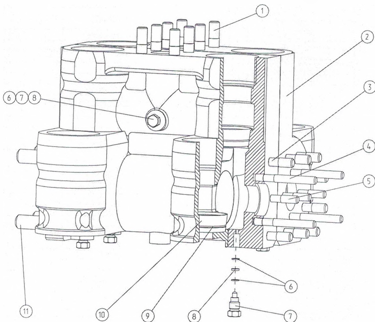
Рисунок 11 - Блок клапанных коробок АФНИ.306555.002
