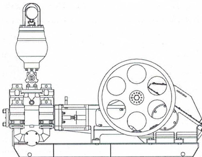
Рисунок 3 - Насос НБ-125ИЖ. Исполнение АФНИ.063168.004-29
