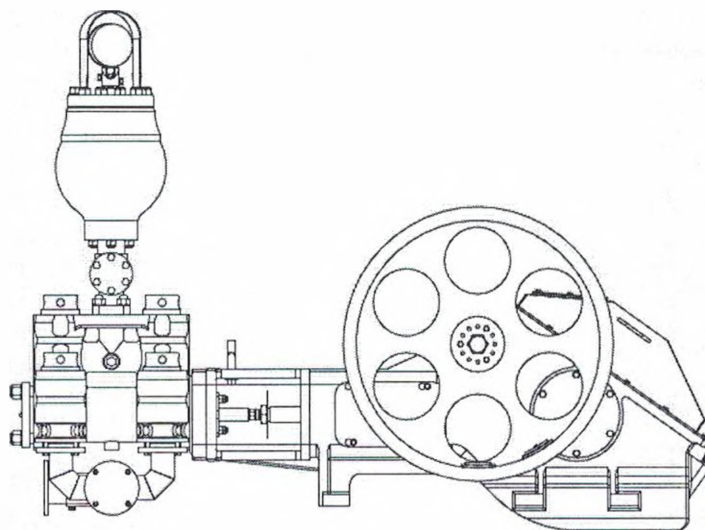
Рисунок 4 - Насос НБ-125ИЖ. Исполнение АФНИ.063168.004-30
