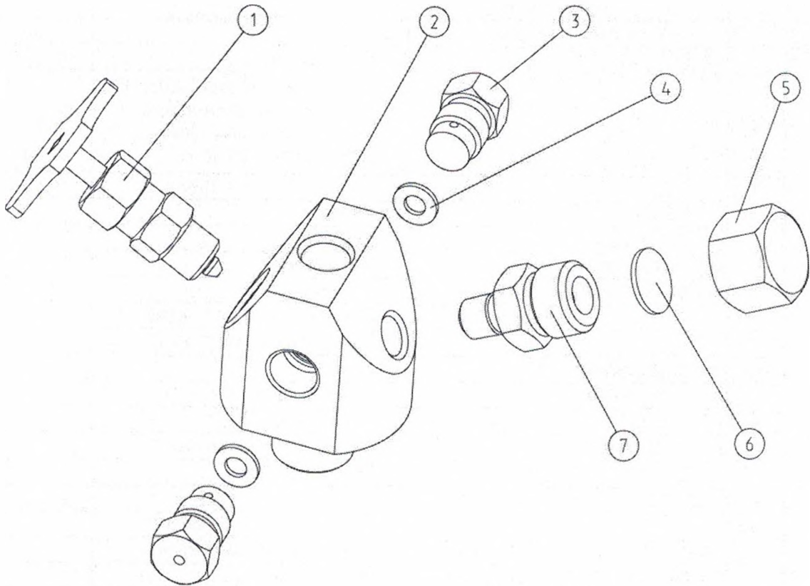
Рисунок 8 - Переходник в сборе КС-10.13.00.000А
