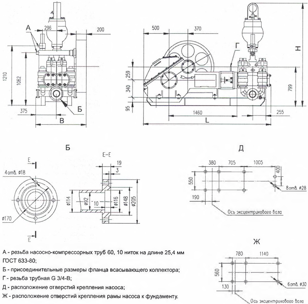
Рисунок 5 - Насос НБ-125ИЖ. Присоединительные размеры
